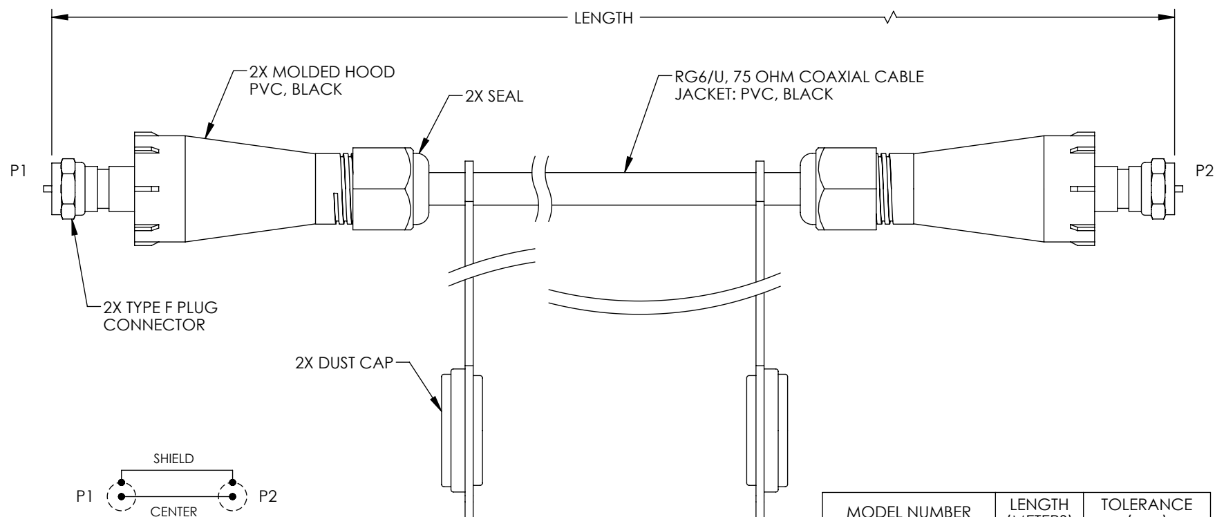
WIRING MAP
