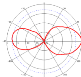
V-Plane: 2450 MHz
