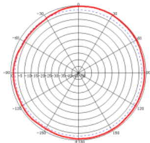
H-Plane: 5100 MHz
