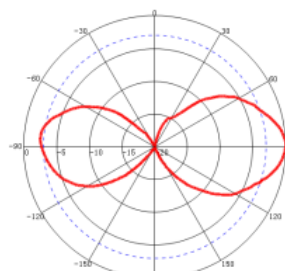
V-Plane: 2500 MHz
