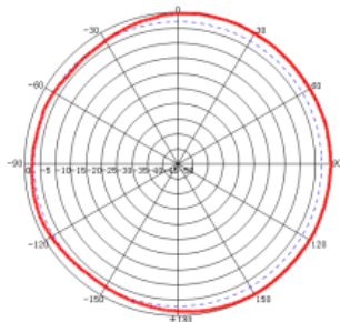
H-Plane: 5500 MHz
