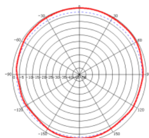
H-Plane: 2450 MHz
