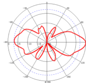
V-Plane: 2400 MHz
