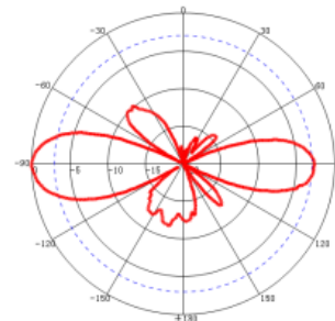
V-Plane: 5100 MHz
