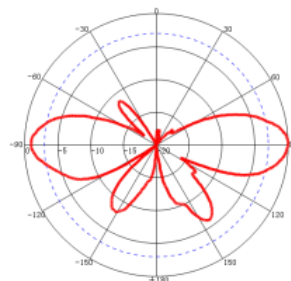
V-Plane: 5100 MHz
