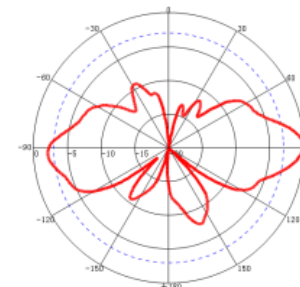
V-Plane: 2450 MHz
