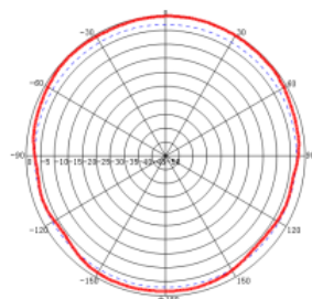
H-Plane: 2400 MHz
