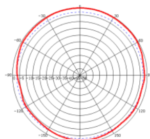
H-Plane: 2500 MHz
