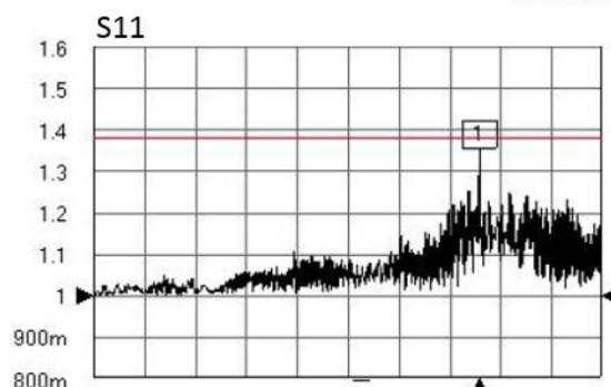
PE3VNA4005-24 VSWR
