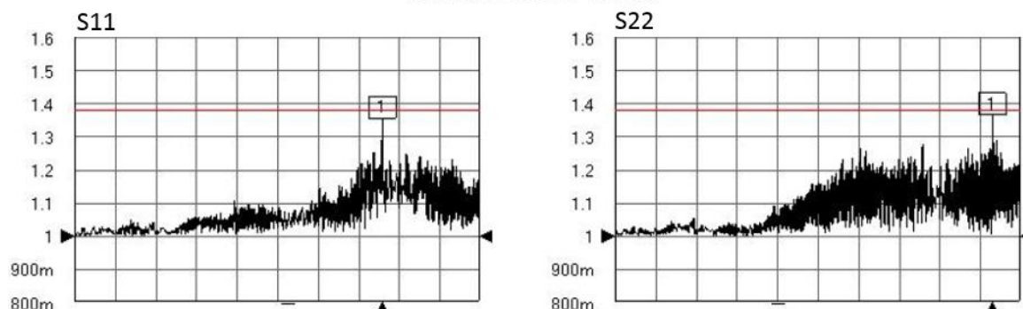
PE3VNA4005-24 VSWR
